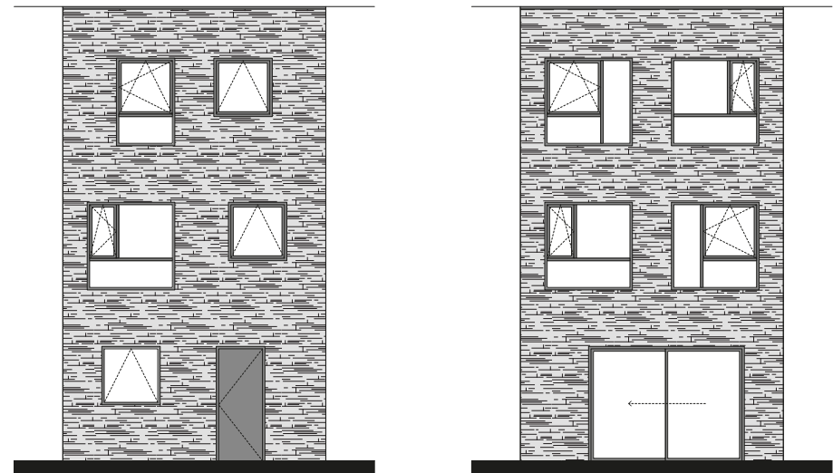
Voor- en achtergevel
