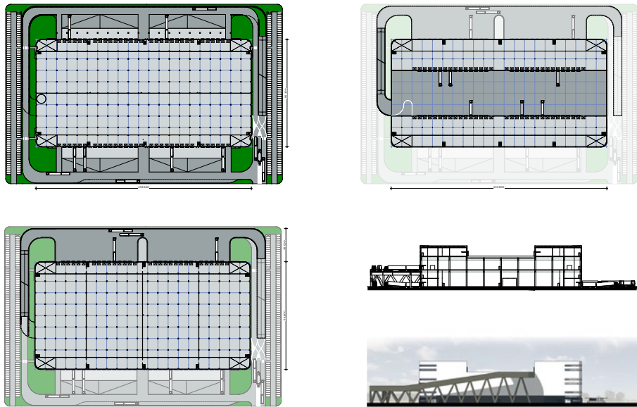
Plattegronden, doorsnede en gevelaanzicht (onder)
